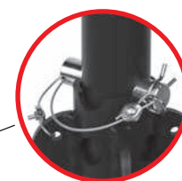
Pasador atado a la base para evitar su pérdida.
