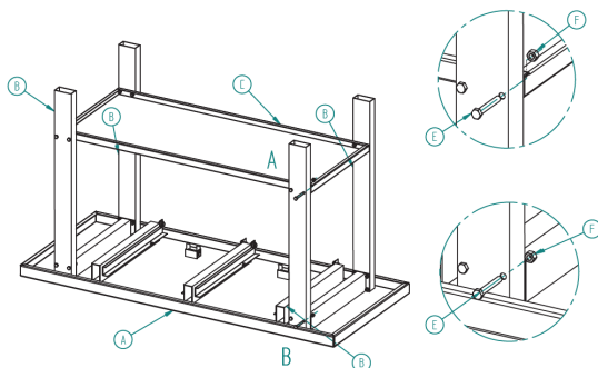
E. Śruba M8X55 (24+1 szt.)
