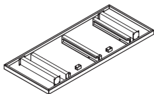
А. Элементы крышки верстака (1 шт.)
