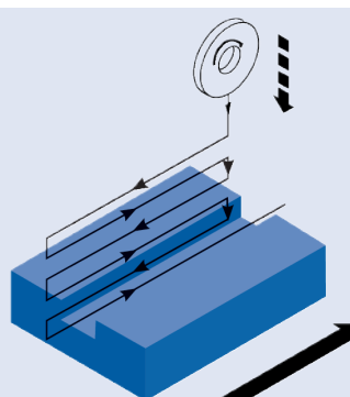
Retificar ranhuras com o avanço no ponto inicial
