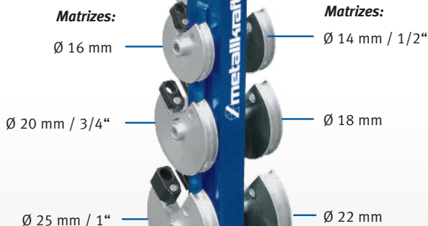
Fig. equipamento de série inclui o conjunto de matrizes Ø 14, 16, 18, 20, 22 e 25 mm
