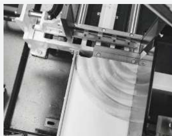
Fenda de corte oscilante para ajuste manual de esquadria
