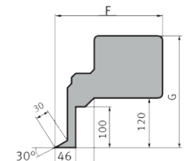
Dimensões mordente HSBM SH
