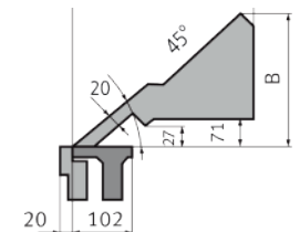
Dimensões mordente HSBM S
