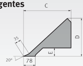
Dimensões mordente HSBM
