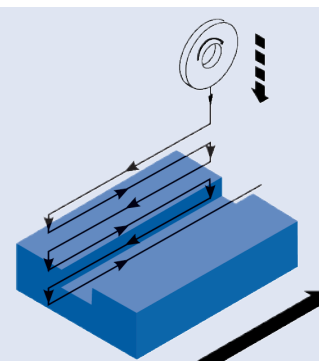
Retificar ranhuras com o avanço no ponto inicial e final
